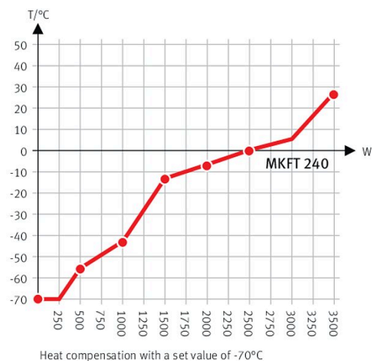
warmtecompensatiediagram
